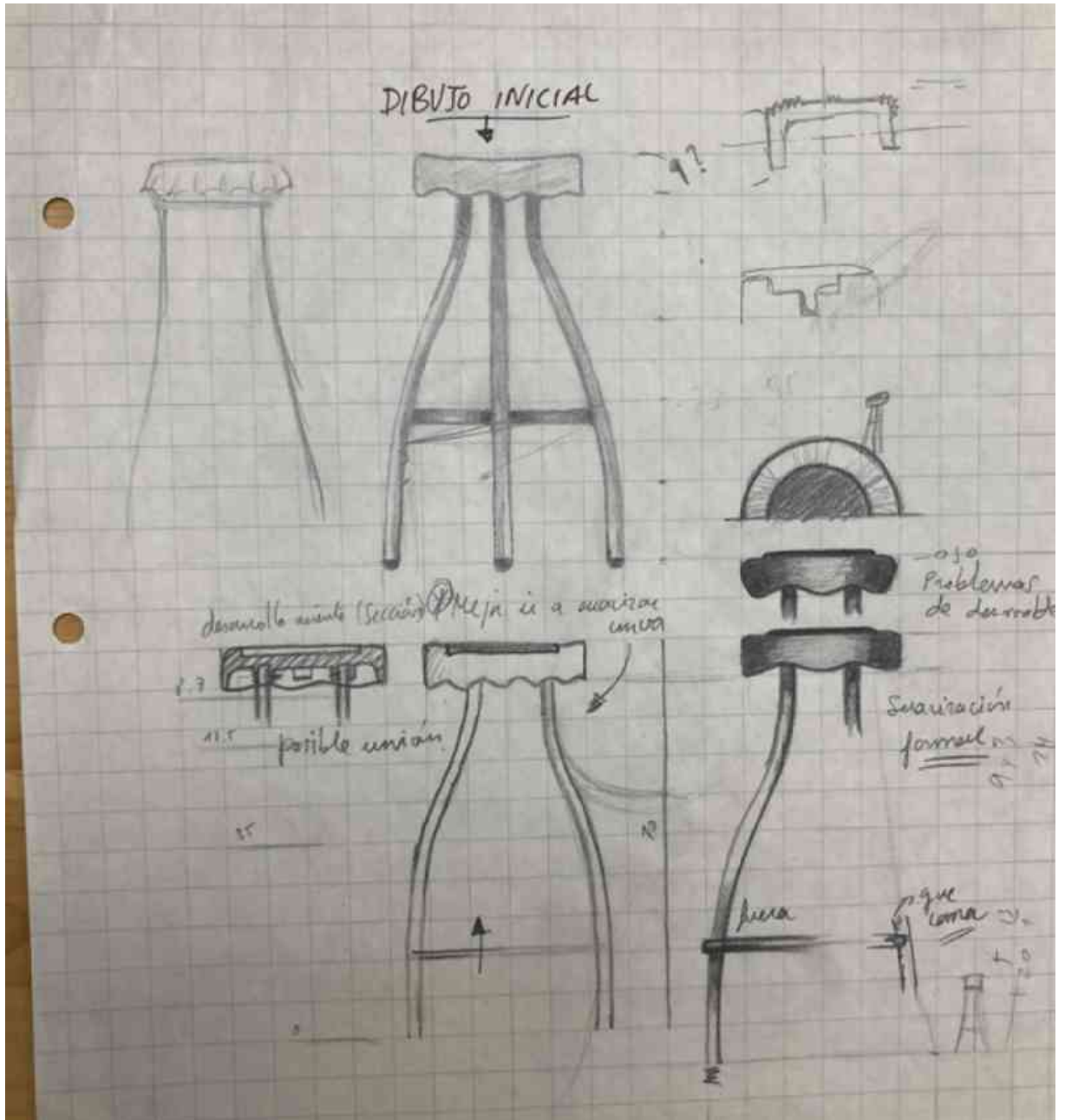
Bocetos iniciales del taburete Bitter , una de las piezas más emblemáticas de la firma Alutec (1998).
